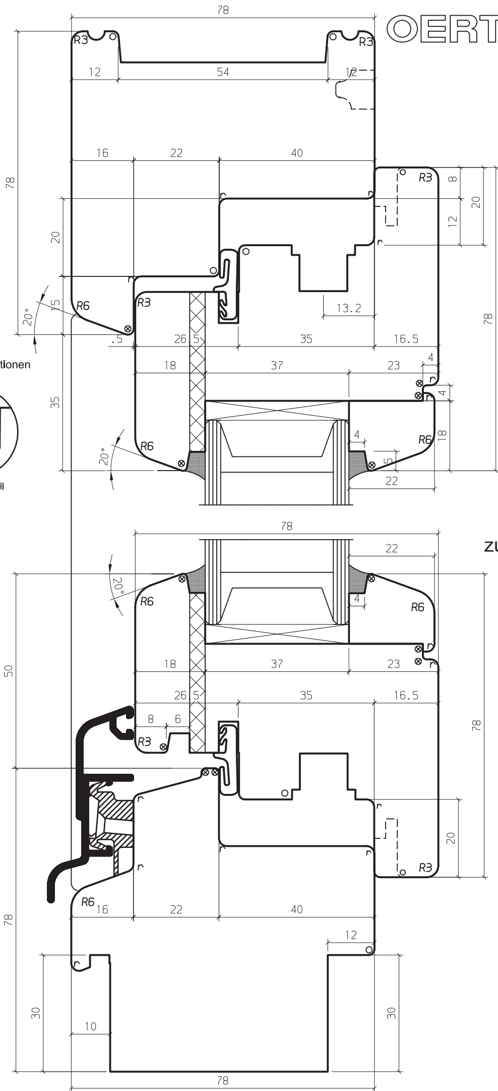
Rahmendichtung (20 mm) bei 12 mm Falzlufte
