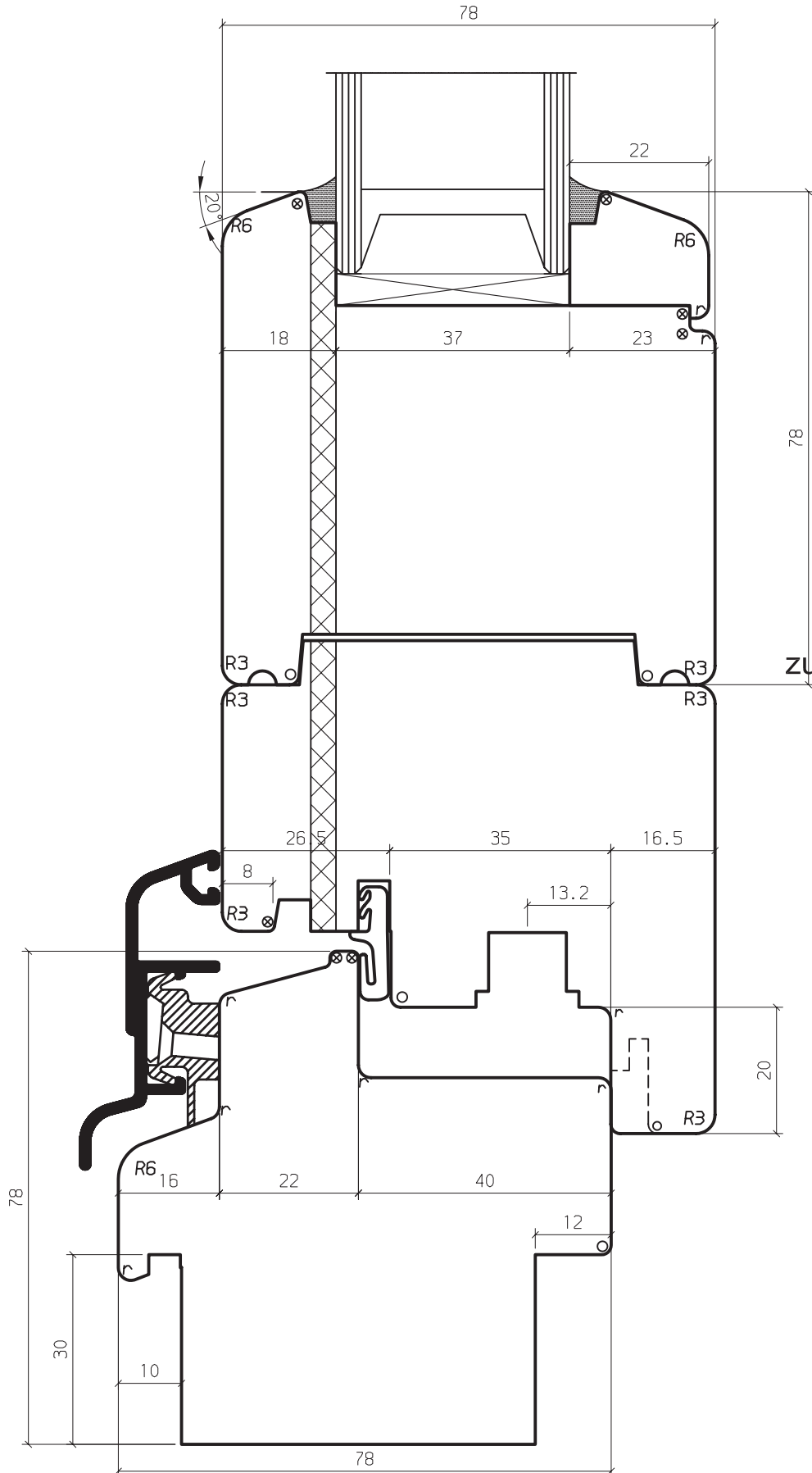
mittlere Überschlagdichtung
